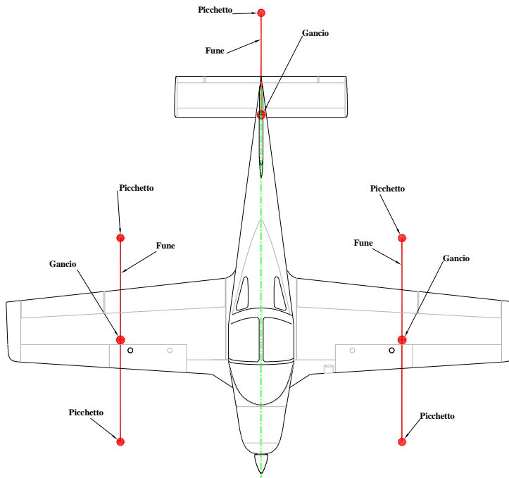
Fig. 8-1. POSIZIONAMENTO DELLE FUNI
