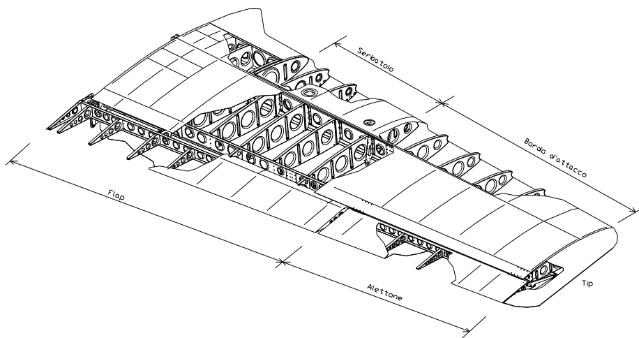
Fig. 7-1. ESPLOSO DELLA SEMIALA DESTRA
