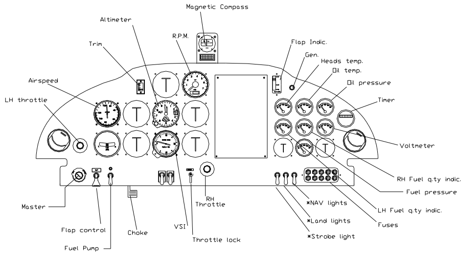
Fig. 7-2. PANNELLO STRUMENTI
