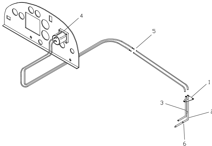
FIG. 7-5. IMPIANTO ANEMOMETRICO
