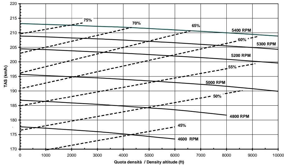
Fig. 5-6 CROCIERA
