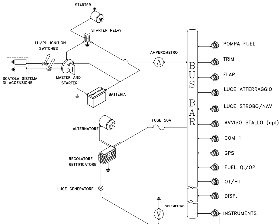
FIG. 7-4. IMPIANTO ELETTRICO
