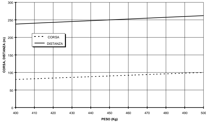
Fig. 5-7 ATTERRAGGIO
